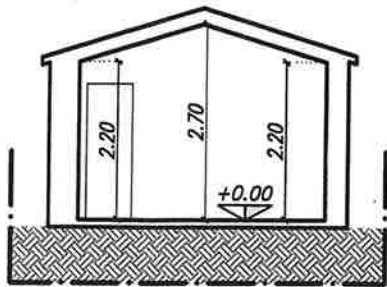
SEZIONE C-C' INARIATA Scala 1:100
