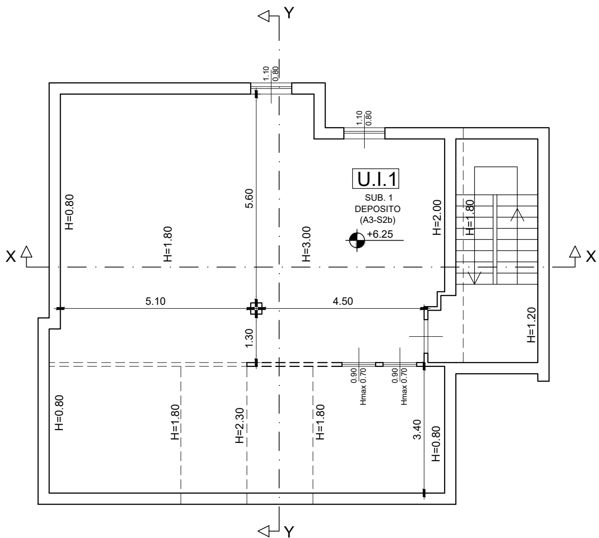
PIANTA PIANO MANSARDATO
